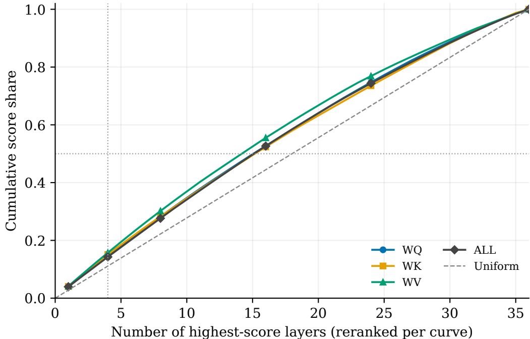
Nonnegative mean KL
