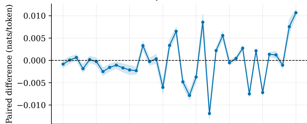
WK - WV: \Delta NLL
