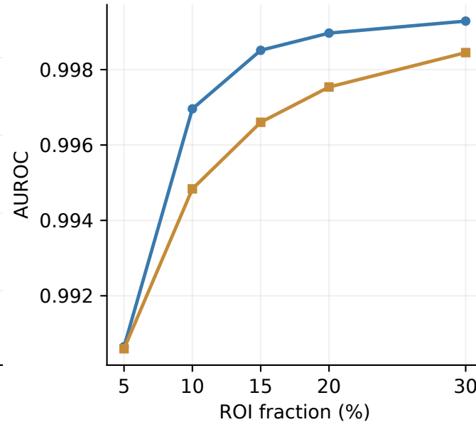
NUAA
