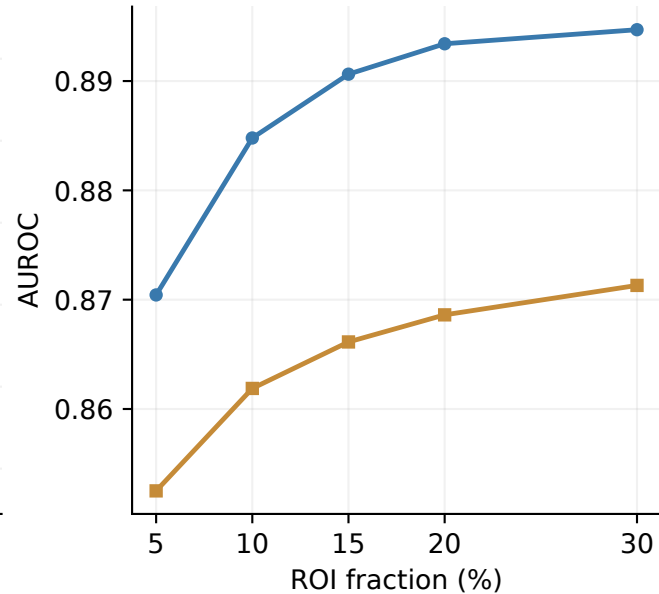
LCC-FASD
