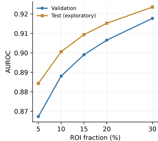
OULU-NPU
