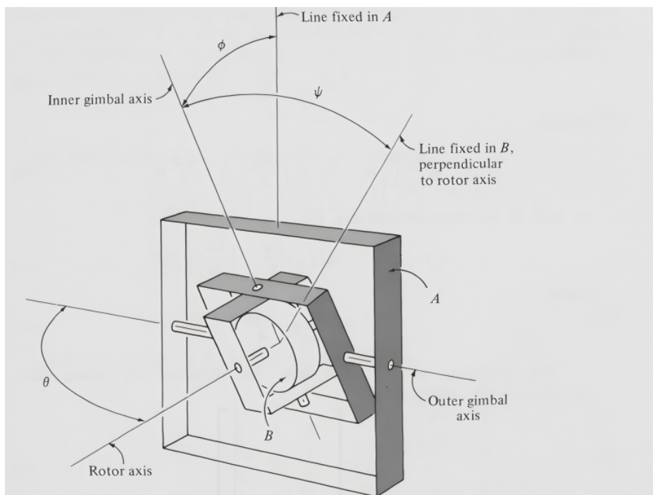
图 3.6: 陀螺转子
