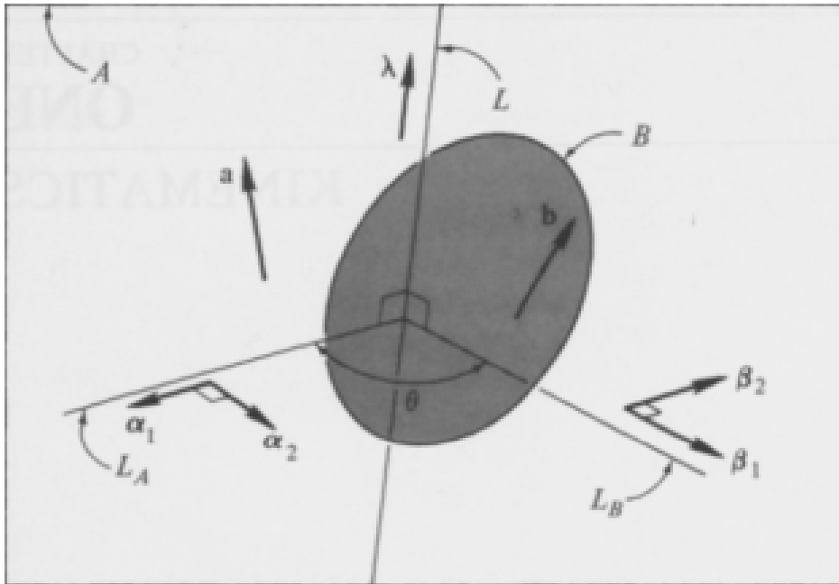
图 3.1: 简单转动
