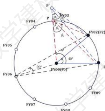
图 7 排布方式 1 的被动机位置
