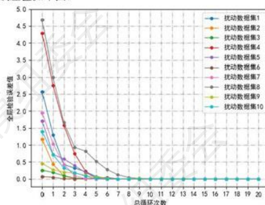
图 28 十组数据集的全局检验误差值
