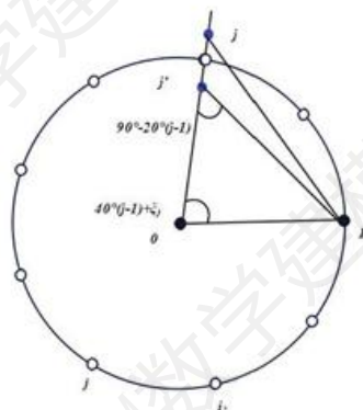
图 12 预处理证明示意图
