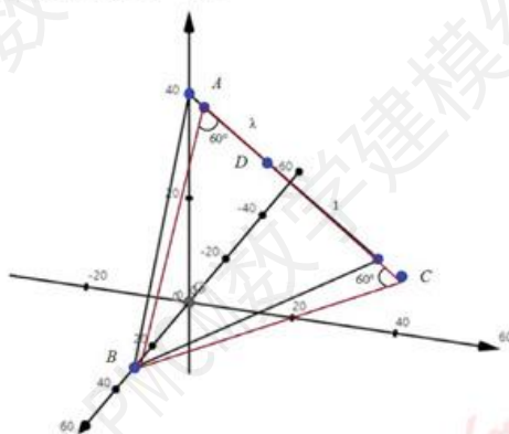
图 21 引理 2 的几何关系
