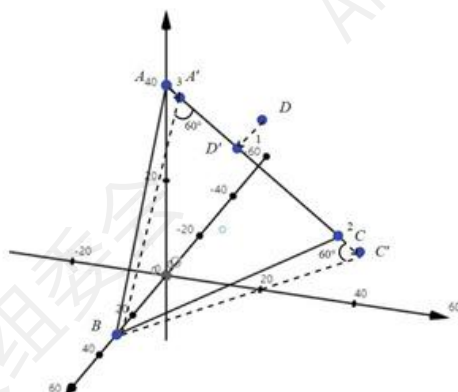
图 20 引理 1 的调整方案
