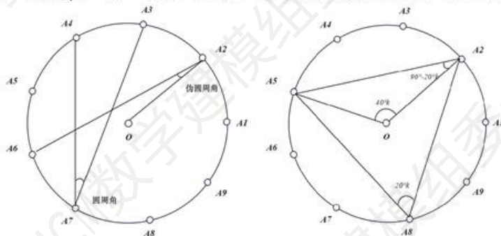
图 8-9 角的定义与引理的证明
