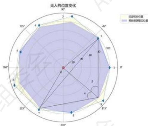
图 16 方案二预处理后的调整图示
