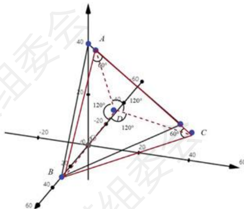
图 22 引理 3 的几何关系
