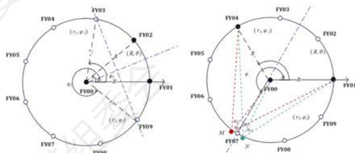
图 4-5 解的几何分布及特殊情况
