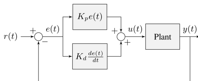
图 3.3: PD 控制器
