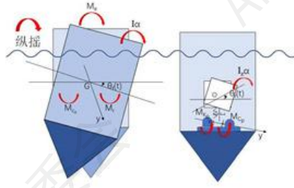
图 10 纵摇运动受力分析示意图
