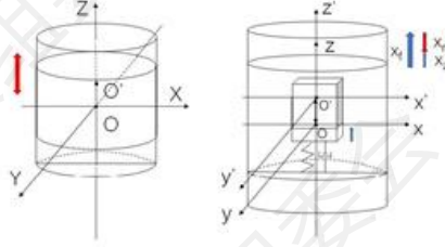
图 1 大地坐标系和固体坐标系示意图
