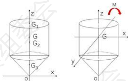
图 11 重心位置确定
