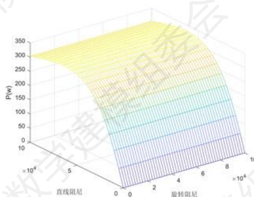
图 13 不同阻尼系数下的功率分布图
