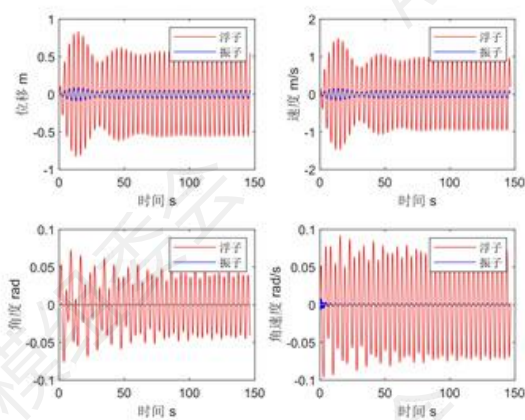
图 12 前 40 周期浮子与振子垂荡和纵摇的（角）位移和（角）速度
