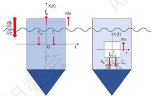
图2 垂荡运动受力分析示意图
