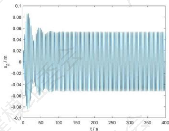
图 8 x_2 关于时间的变化
