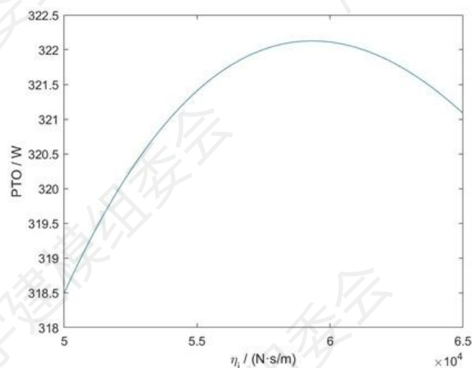
图 13 PTO 关于 \eta_l 的局部遍历图
