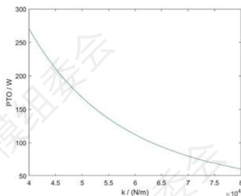
图 18 弹簧刚度的稳定性分析图
