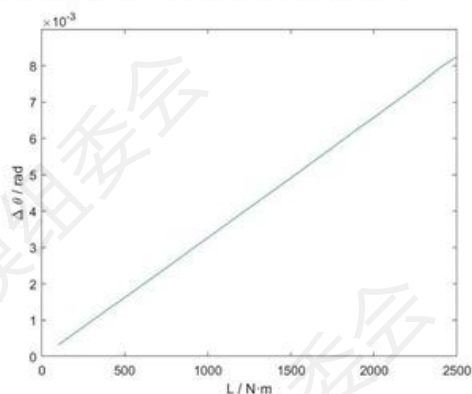
图 16 波浪激励力矩的稳定性分析图
