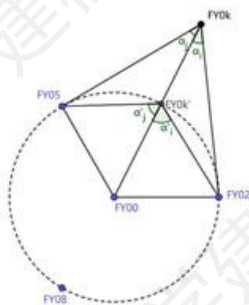
图 7-3 长度坐标调整示意图
