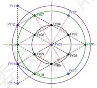
图 8-1 锥形编队圆形化分类示意图
