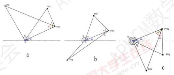
图 5-1 相对位置关系图-1
