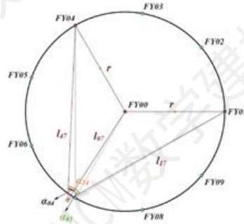
图 1: 三架无人机无源定位示意图
