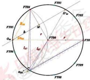
图 5: 圆心坐标的求解
