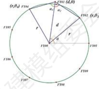
图 2: 正弦定理求解坐标
