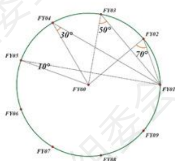
图 6: 标准位置角度 (1)
