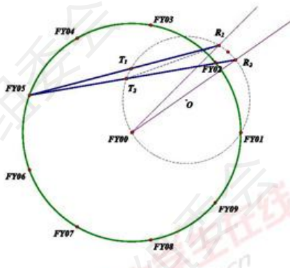
图 11: 角度误差证明示意图
