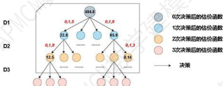
图 14: 决策树示意图
