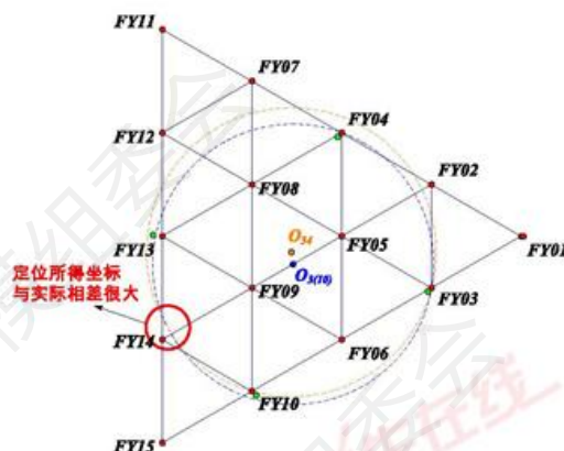
图 17: 四点共圆情况示意
