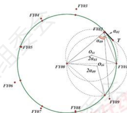
图 13: 确定初始点坐标
