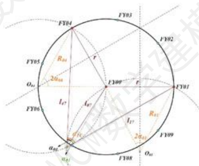
图 4: 等角对等边示意图
