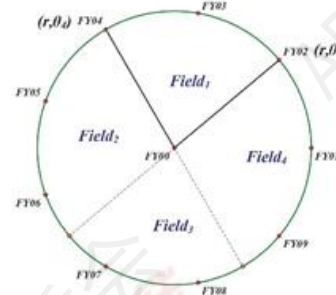
图 3: 正弦定理求解坐标的局限性
