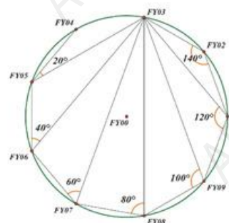
图 7: 标准位置角度 (2)
