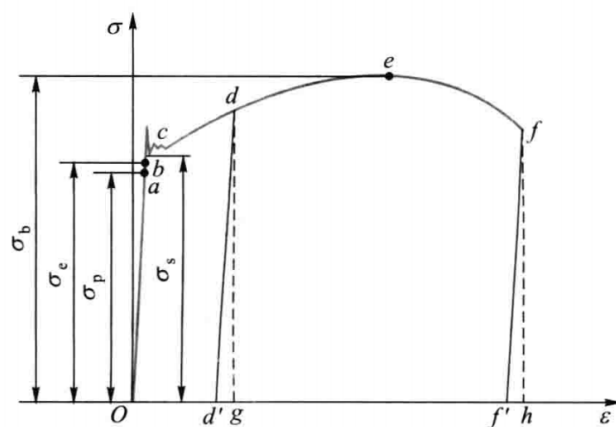
图 2.2: 低碳钢拉伸时的 \sigma - \epsilon 曲线
