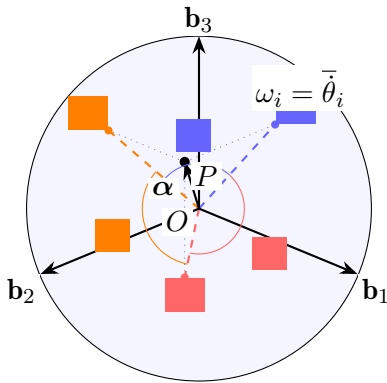
图 3.11: 角速度分量的几何解释: \omega_i 等于夹角 \theta_i 的时间导数在单位球面上的空间平均值, 即 \omega_i = \bar{\dot{\theta}}_i ( i = 1, 2, 3 )。图中 \beta_i 为固定在 A 中的单位向量 \boldsymbol{\alpha} 在垂直于 \mathbf{b}_i 的平面上的正交投影。
