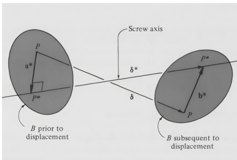
图 3.9: 螺旋运动
