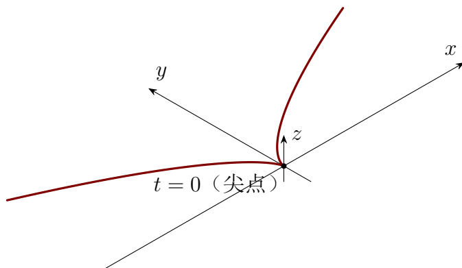
图 2.2: 半立方抛物线 \mathbf{r}(t) = (t^3, t^2, 0)
