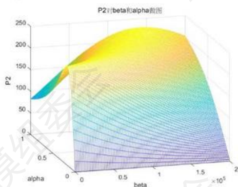
图 8 P 对 \beta 和 \alpha 作图
