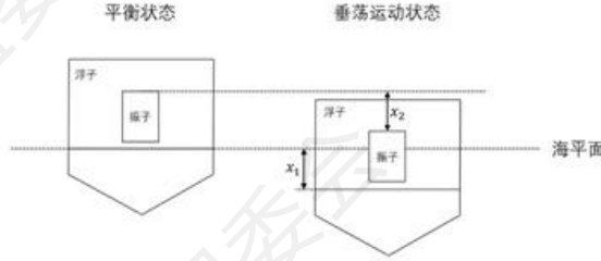
图 1 浮子坐标示意图
