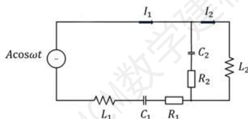
图 6 力电比拟等效电路图
