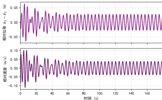
问题1. (1): 直线阻尼系数为常数时的垂荡位移和速度
