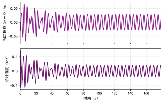
问题1. (2): 阻尼系数随相对速度变化时的垂荡位移和速度
