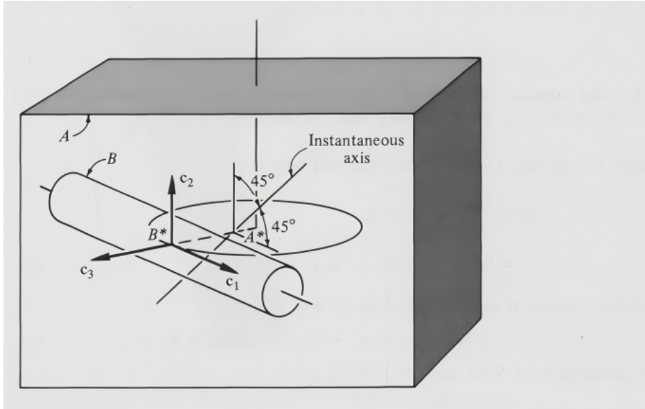
图 3.16: 瞬时轴例题
