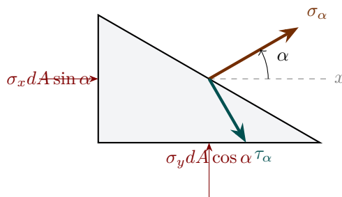
图 9.1: 二向应力状态隔离体受力分析
