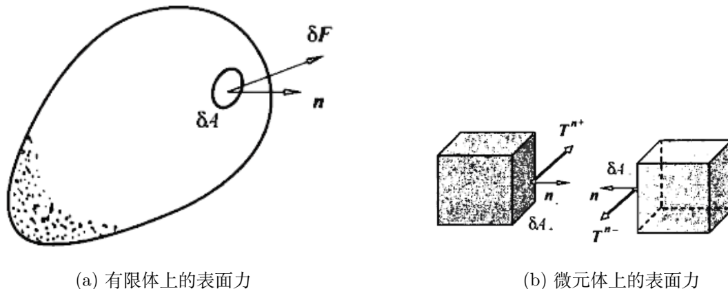
图 3.1: 流体中表面力的示意图
