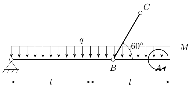
图 A-2 复习题 2 结构简图 (据原稿重绘)
