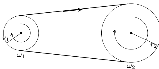
图 7.6: 带传动：带与轮缘间不打滑时，两轮边缘处带的线速度相等
