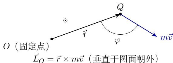
图 12.1: 质点对固定点的动量矩
