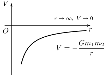
图 13.3: 万有引力场的势能示意：以无穷远处为零势能点， V = -\frac{Gm_1m_2}{r}
