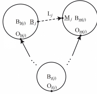
图 9.3: 切断铰及其关联的体元
