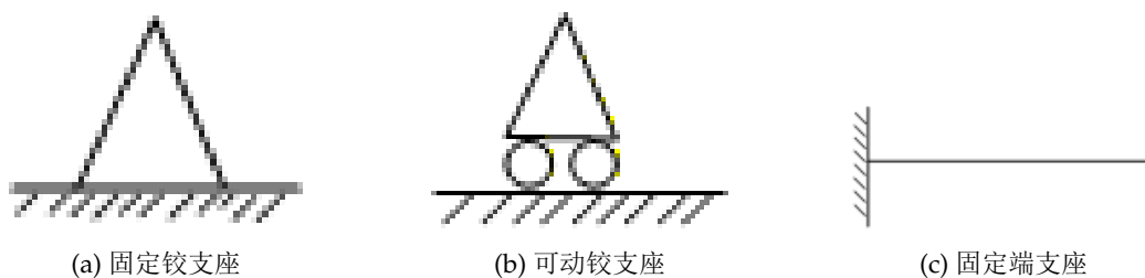
图 5.1: 支座示意图
