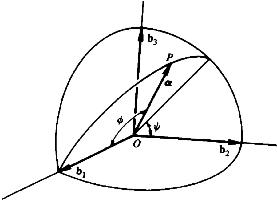
图 3.13: 角速度分量: 单位球面上的 \phi 与 \psi
