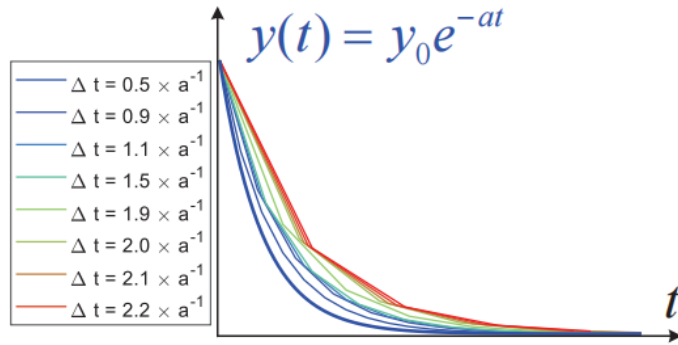
图 2.3: 向后欧拉法：不同步长 \Delta t 下的数值解对比（绝对稳定）
