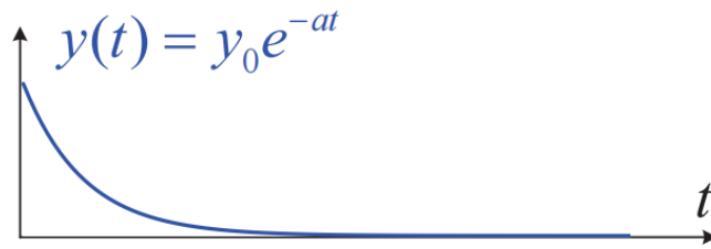
图 2.1: y(t) = y_0 e^{-at} 指数衰减解析解
