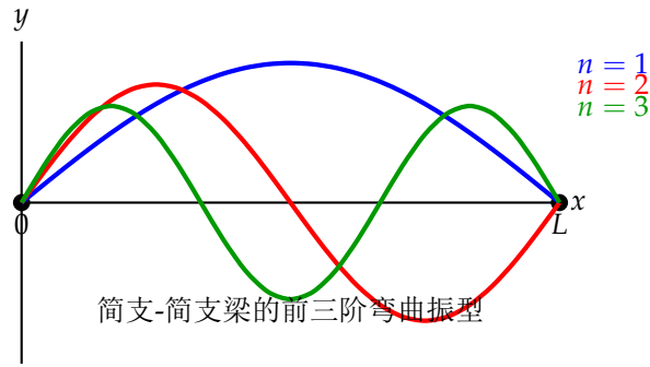
图 8.2: 简支梁的前三阶弯曲振型。与弦的振型形式相同（正弦函数），但频率与 n^2 成正比
