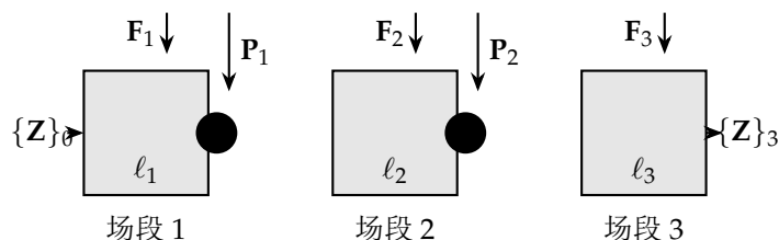
图 9.3: 传递矩阵法的链式结构模型。场段通过场矩阵 \mathbf{F} 传递，集中元件通过点矩阵 \mathbf{P} 连接
