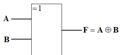
图 2.7: 异或门逻辑符号
