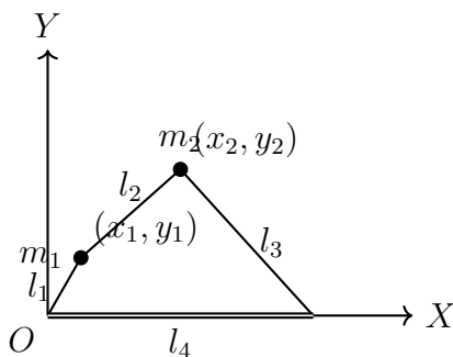
图 5.1: 平面四连杆机构
