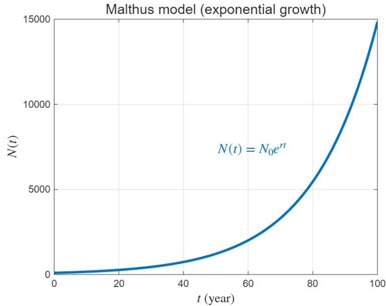
图 1.3: Malthus 人口模型的指数增长曲线。MATLAB 代码见 MATLAB 代码/Malthus 人口模型.m。
