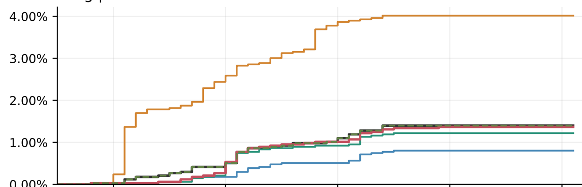
Object | Cumulative FPR
