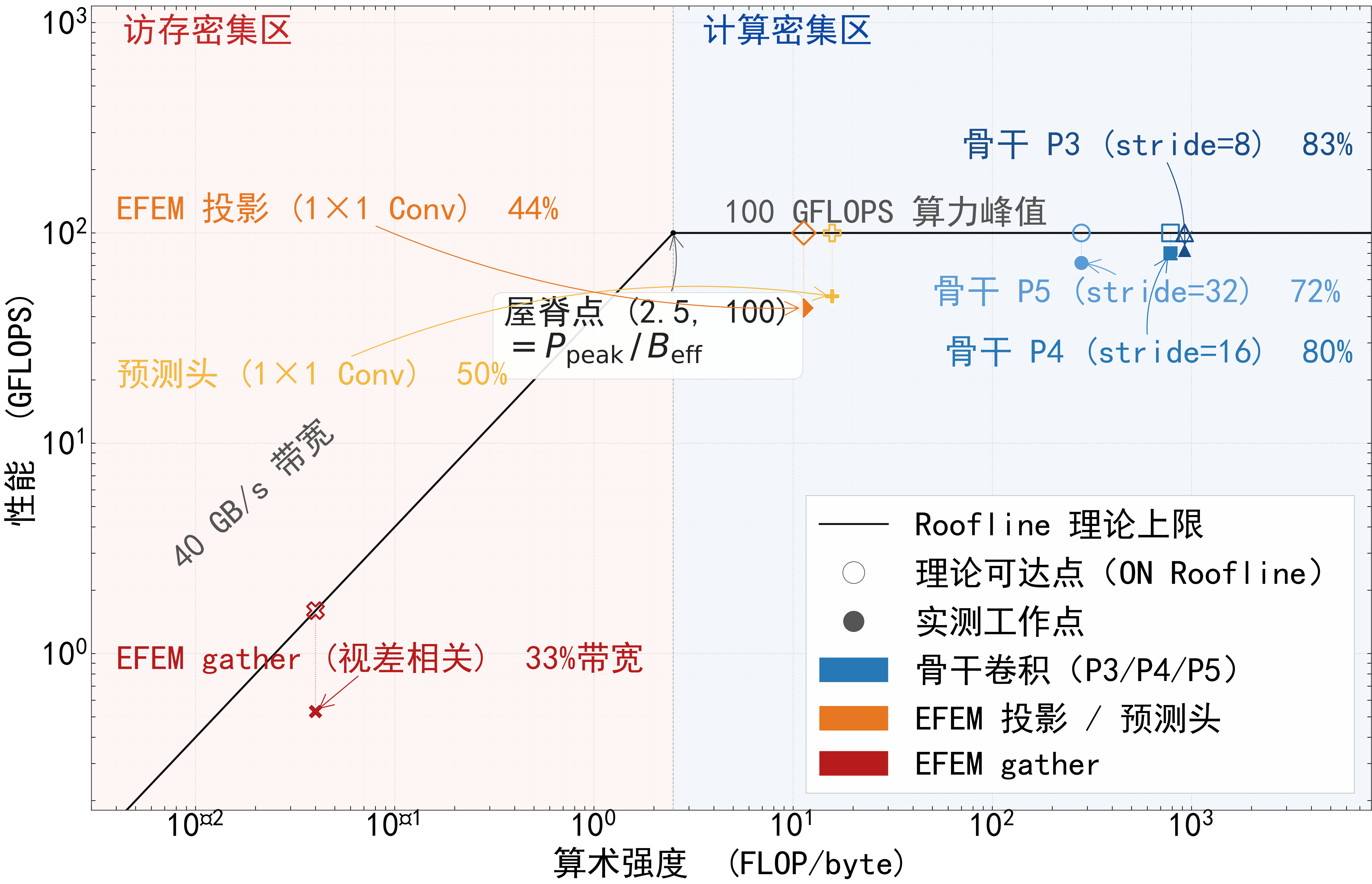
骁龙 8 Gen3 CPU Roofline 模型 (FP16, 4 线程, batch = 1)
