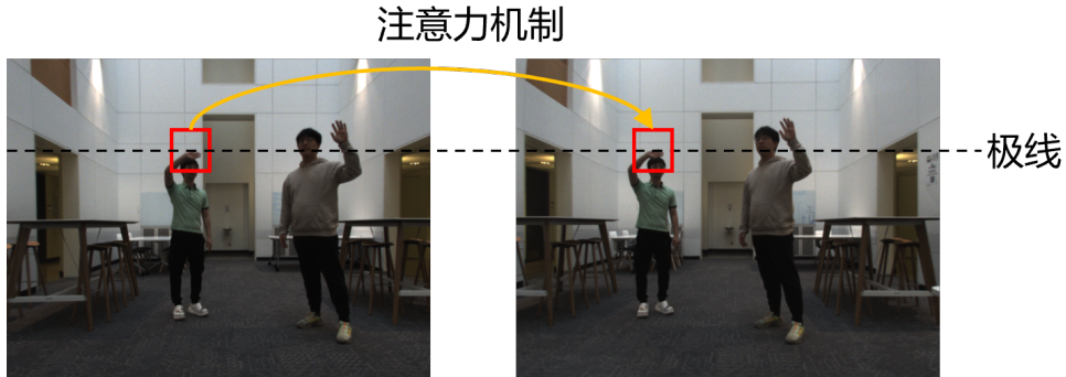
图 3-4 极线交叉注意力计算示意图：右视图特征作为 Query，左视图特征作为 Key/Value，沿水平极线在视差窗口内计算权重并对 Value 加权聚合。
