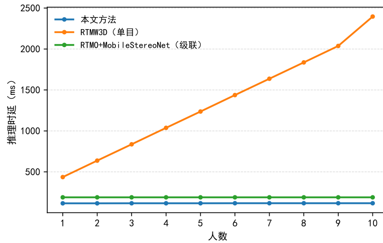
图 3-6 端侧推理时延随人数变化的对比（数据来自 StereoMulti3DPose 的 Xiaomi 14/MNN/FP16/4-thread 测量）。
