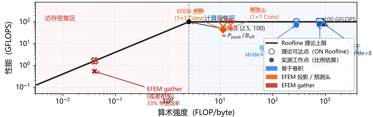
骁龙 8 Gen3 CPU Roofline 模型 (FP16, 4 线程, batch = 1)
