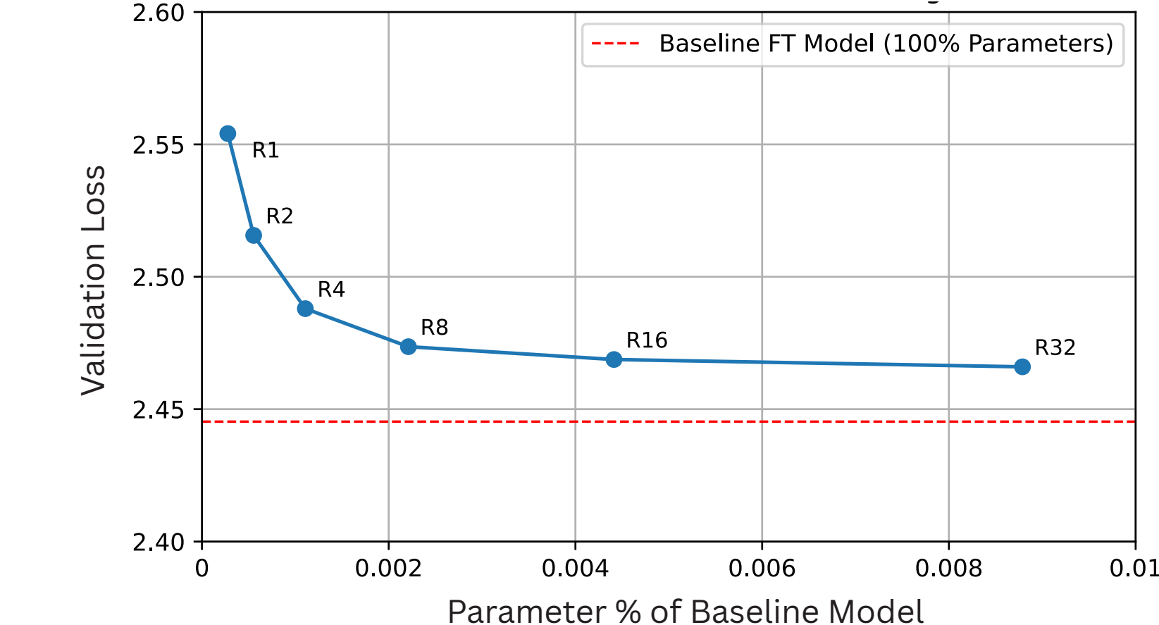
Validation Loss vs Parameter %
