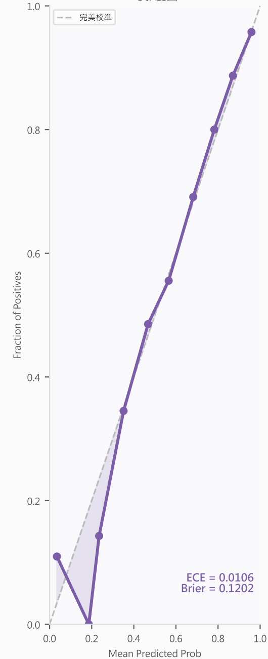
可靠度圖
