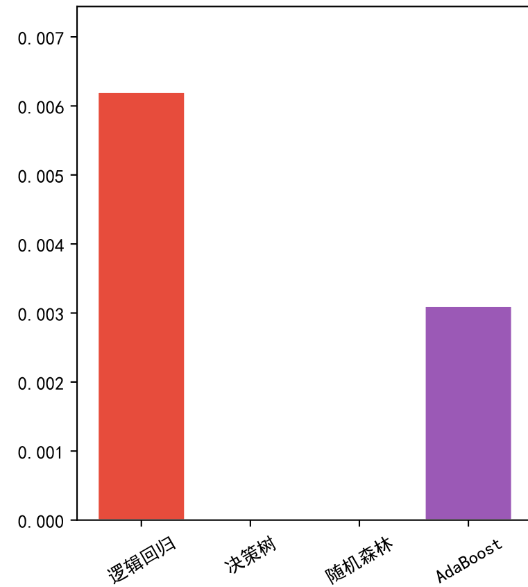
F1
