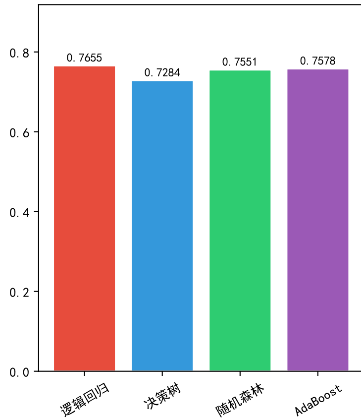
测试集AUC
