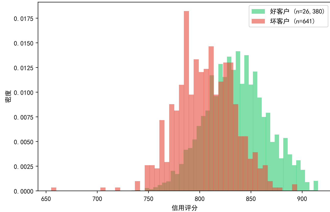
好/坏客户评分分布
