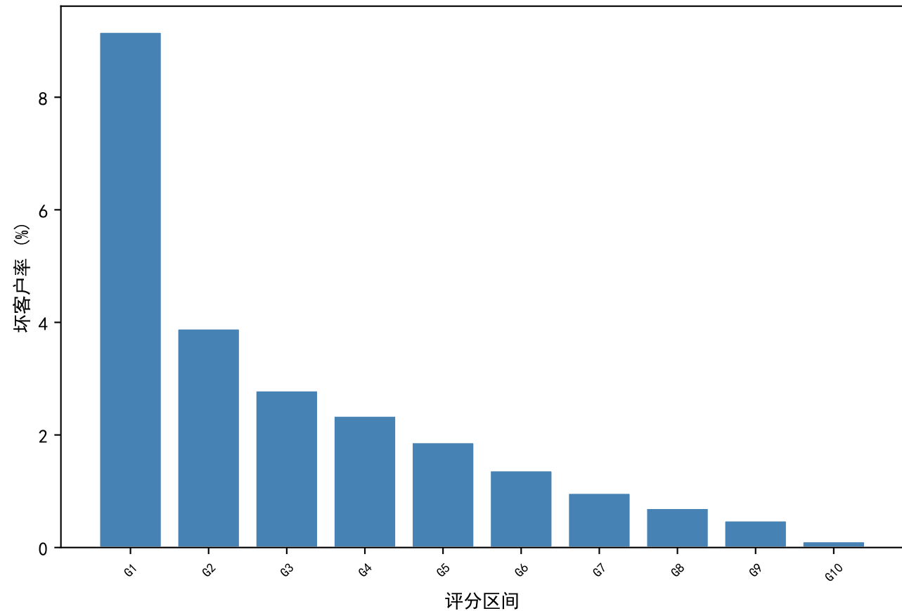
各评分区间坏客户率
