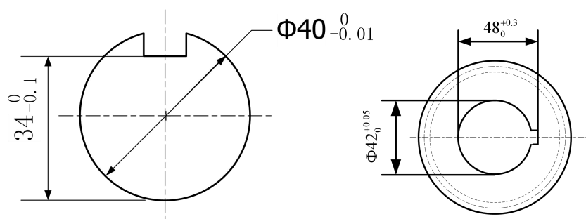
a 零件图
