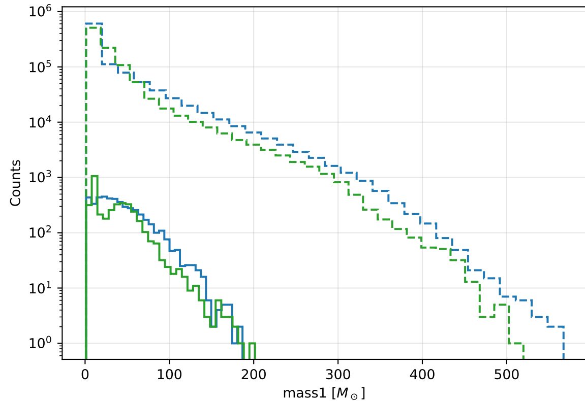
GWTC-3 vs GWTC-4: Mass1
