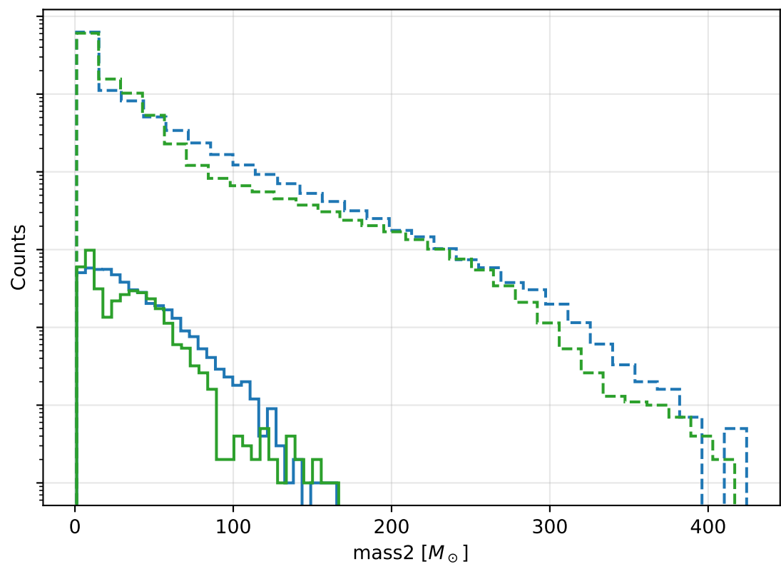
GWTC-3 vs GWTC-4: Mass2
