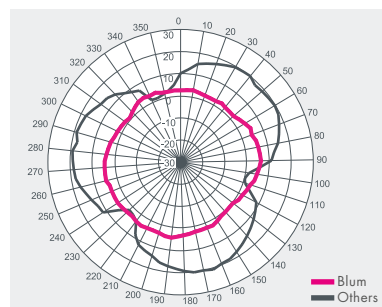
无圆周凸角的接触测量特性
