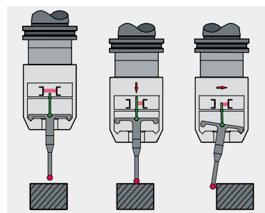
先进的光电式信号触发原理·精度极高
