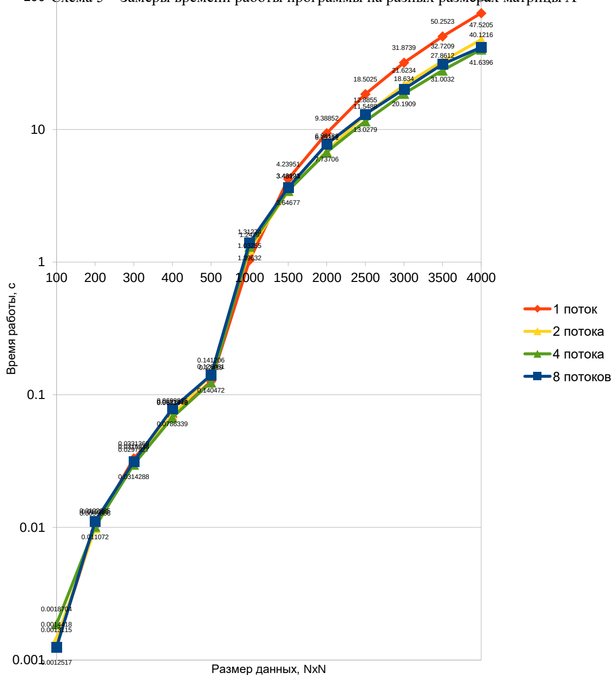
100 Схема 5 – Замеры времени работы программы на разных размерах матрицы A
