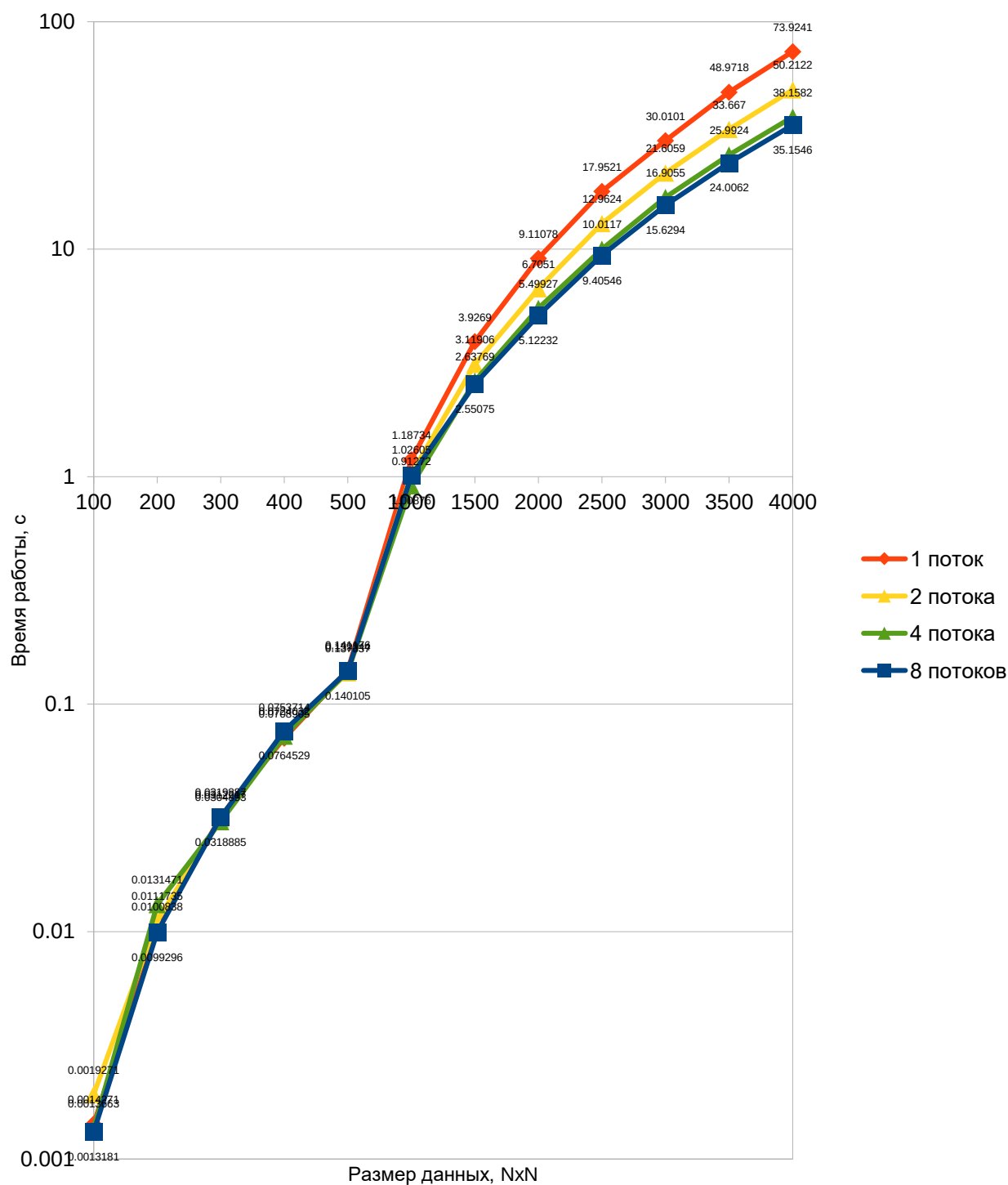
Схема 6 – Замеры времени работы программы на разных размерах матрицы A
