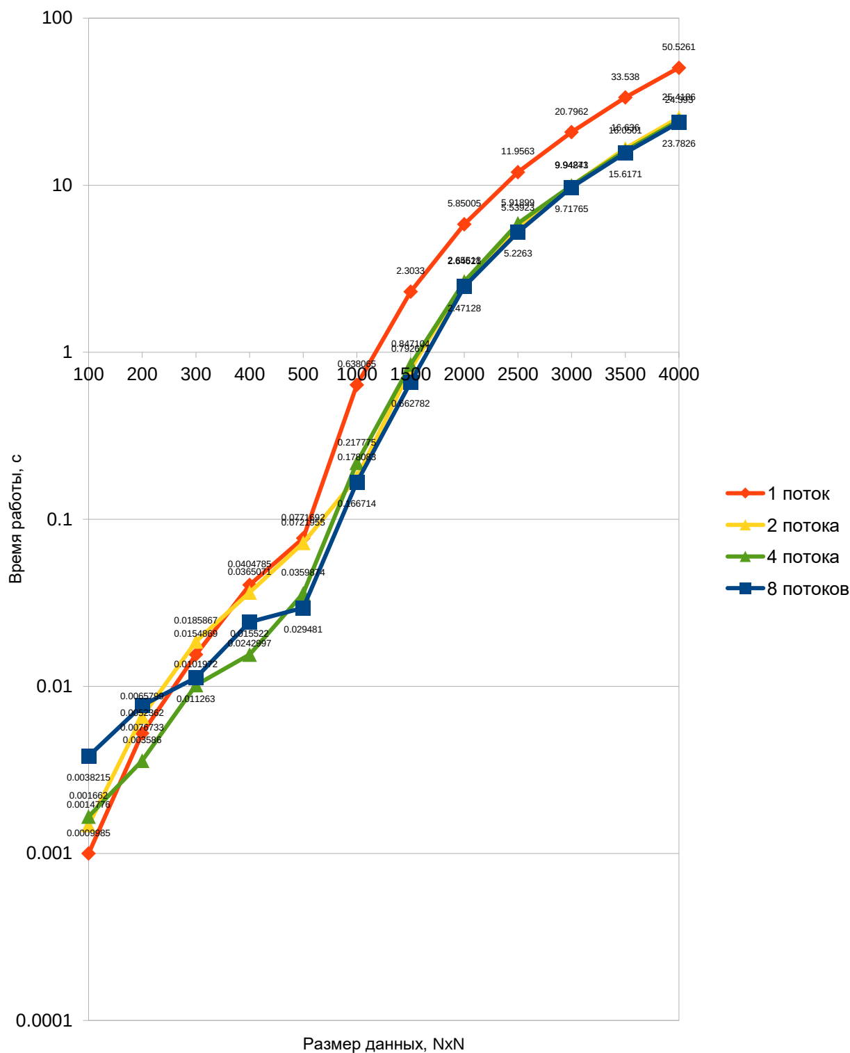
Схема 3 – Замеры времени работы программы на разных размерах матрицы A
