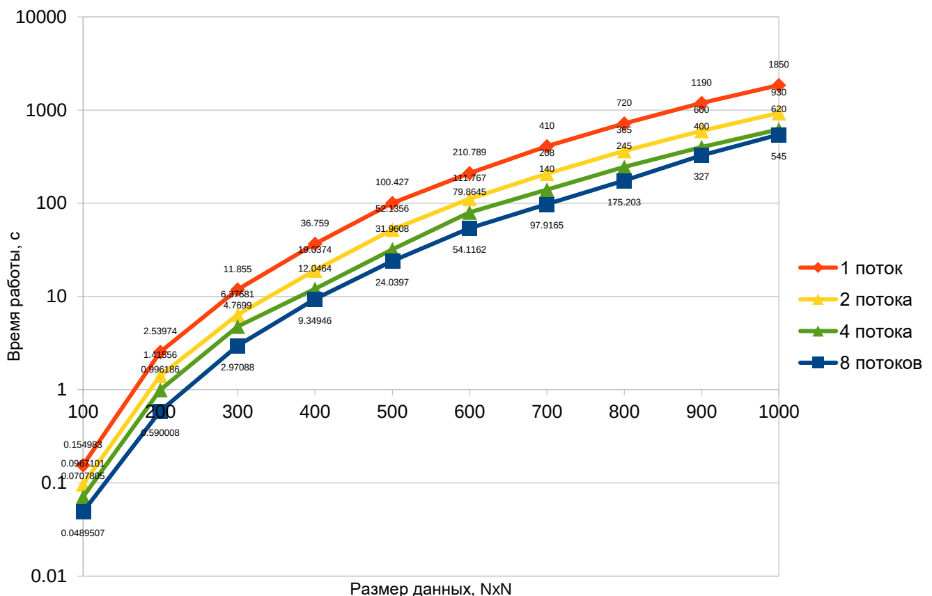
Схема 1 – Замеры времени работы программы на разных размерах матрицы A
