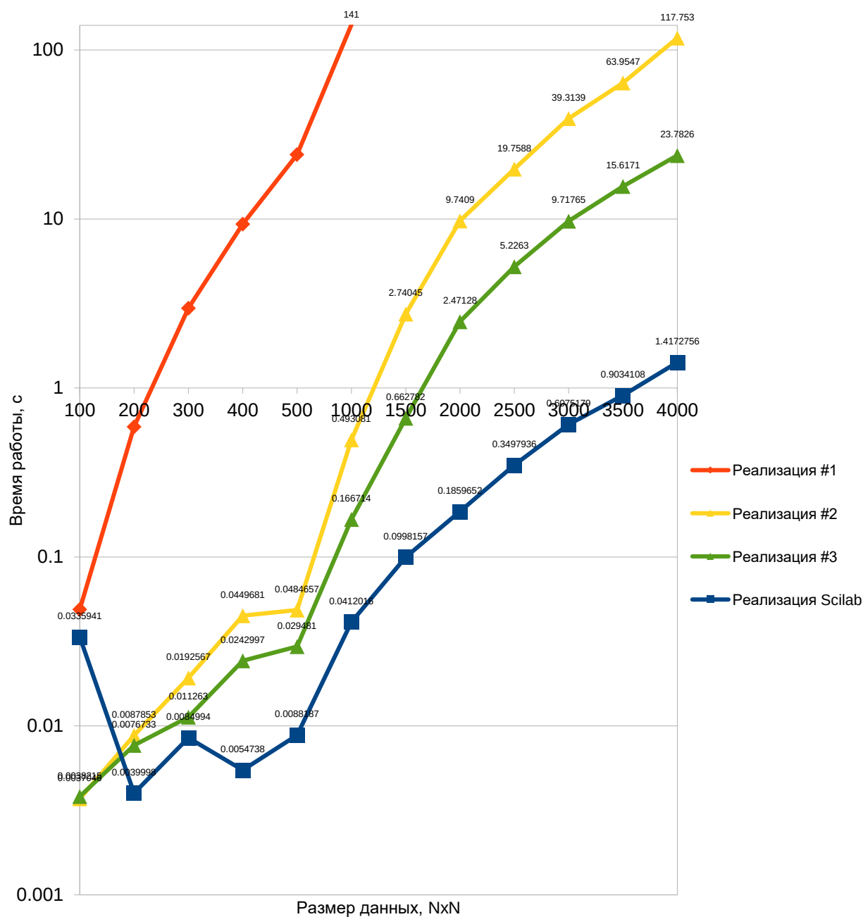
Схема 4 – Сравнение реализаций QR-разложения методом Хаусхолдера с QR-разложением из библиотеки SciLab
