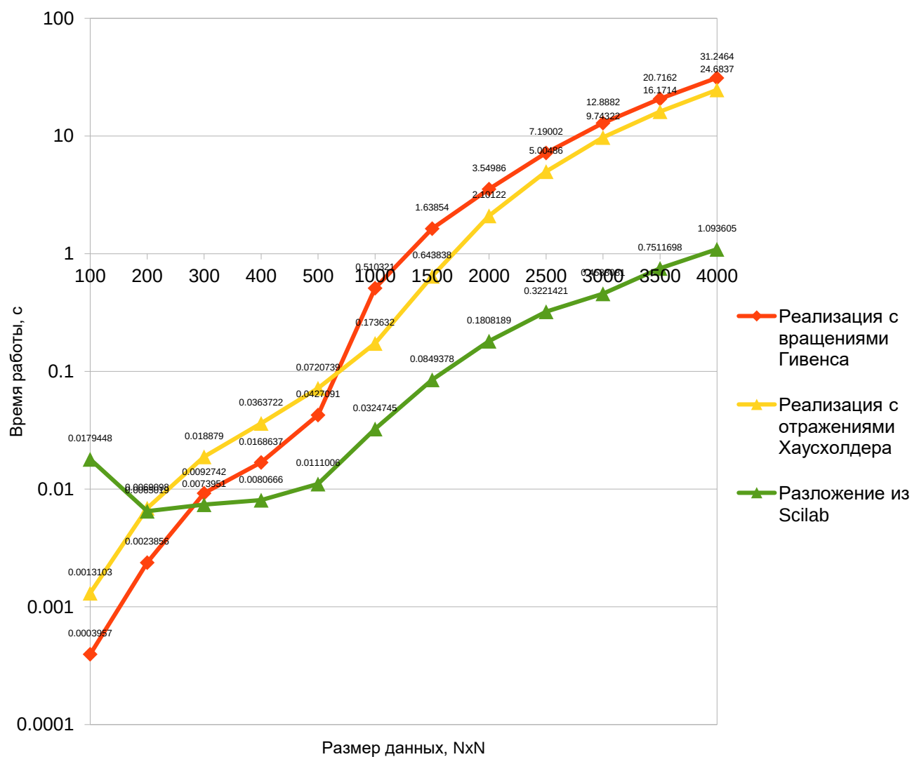
Схема 10 – Сравнение скорости решения QR-разложения нижней хессенберговой матрицы методом Гивенса, методом Хаусхолдера и QR разложением из библиотеки SciLab
