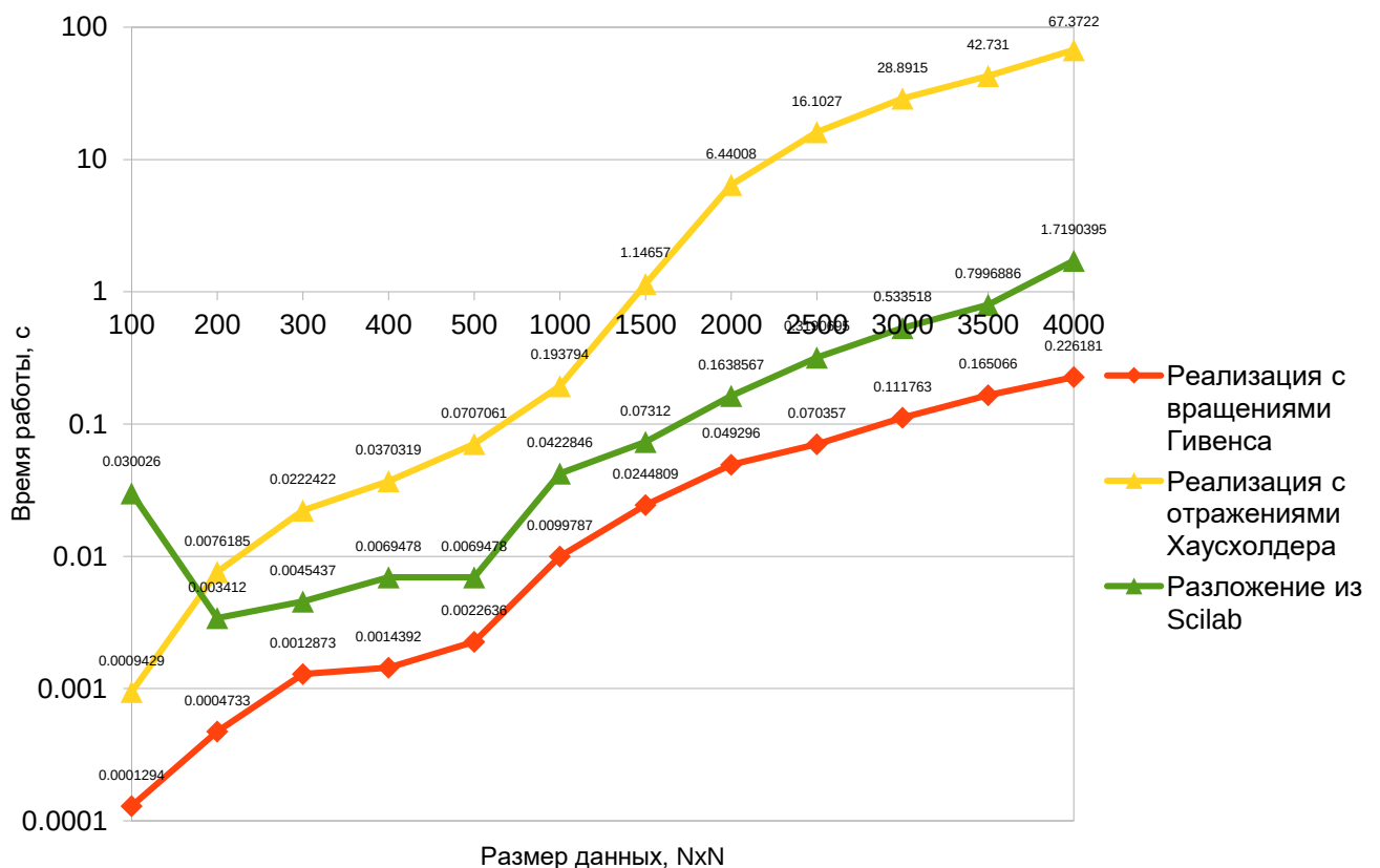
Схема 9 – Сравнение скорости решения QR-разложения верхней хессенберговой матрицы методом Гивенса, методом Хаусхолдера и QR разложением из библиотеки SciLab
