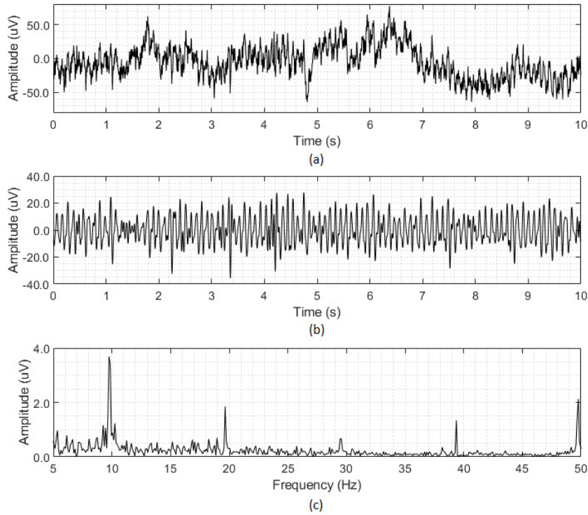
Rysunek 2.3: Przykład SSVEP użytkownika patrzącego na bodziec migający z częstotliwością 10 Hz: EEG w dziedzinie czasu (a); EEG po filtracji w dziedzinie czasu (b); EEG w dziedzinie częstotliwości (c). Źródło: [o].
