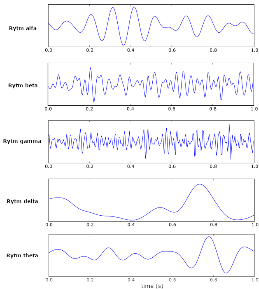
Rysunek 1.3: Próbkki sygnałów poszczególnych rytmów EEG [o]
