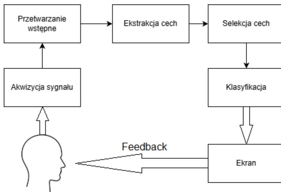
Rysunek 1.1: Schemat struktury interfejsu mózg-komputer (Źródło: opracowanie własne na podstawie [o])
