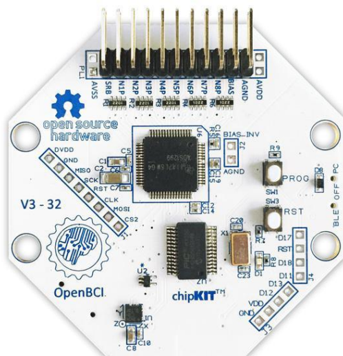
Rysunek 3.2: Urządzenie OpenBCI Cyton wykorzystane w eksperymencie. Źródło: [o]
