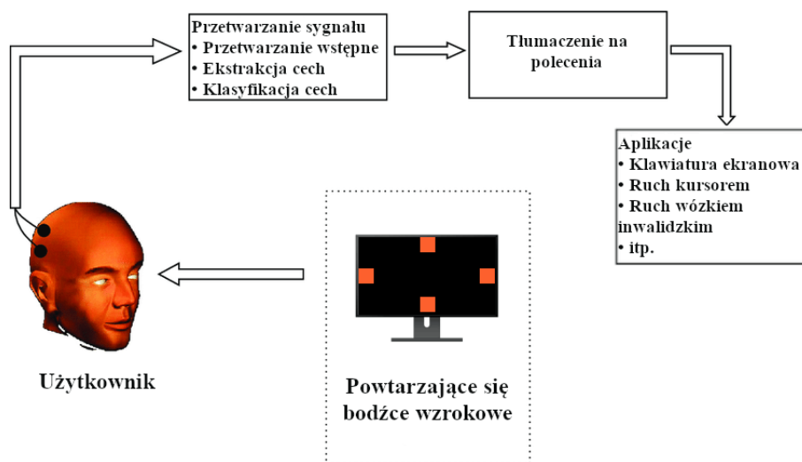
Rysunek 2.1: Funkcjonalny model interfejsu BCI opartego na SSVEP. Opracowanie własne na podstawie: [0].
