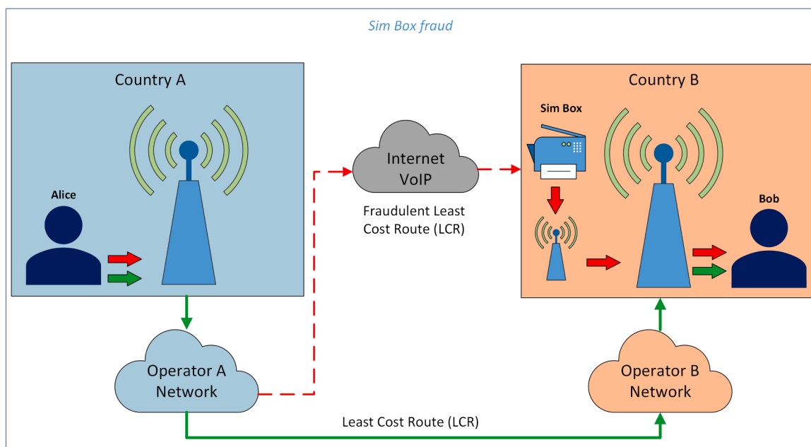
Fig. 3. SIM Box fraud.
