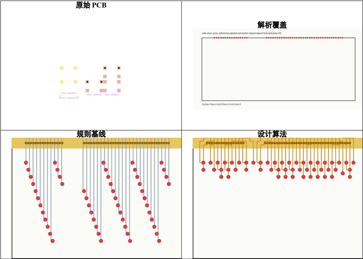
图 A-6 mini pcie reference 案例独立截图对比
