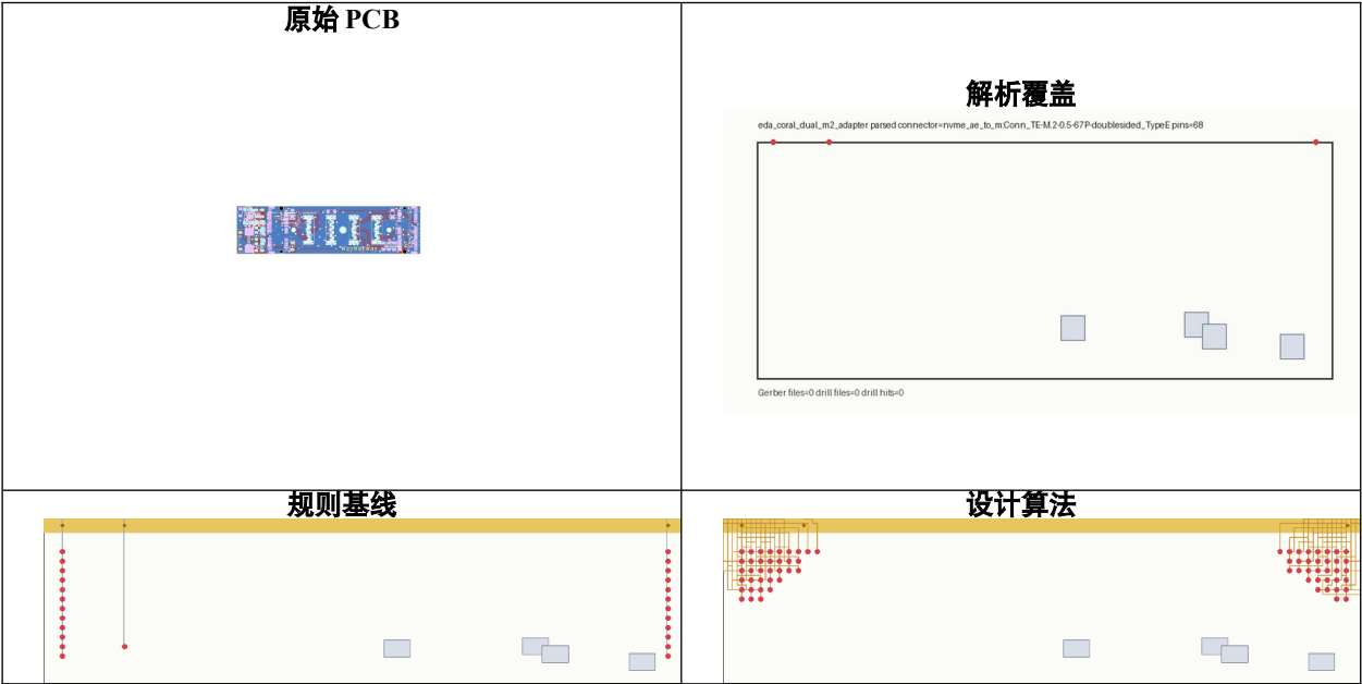
图 A-7 coral dual m2 adapter 案例独立截图对比
