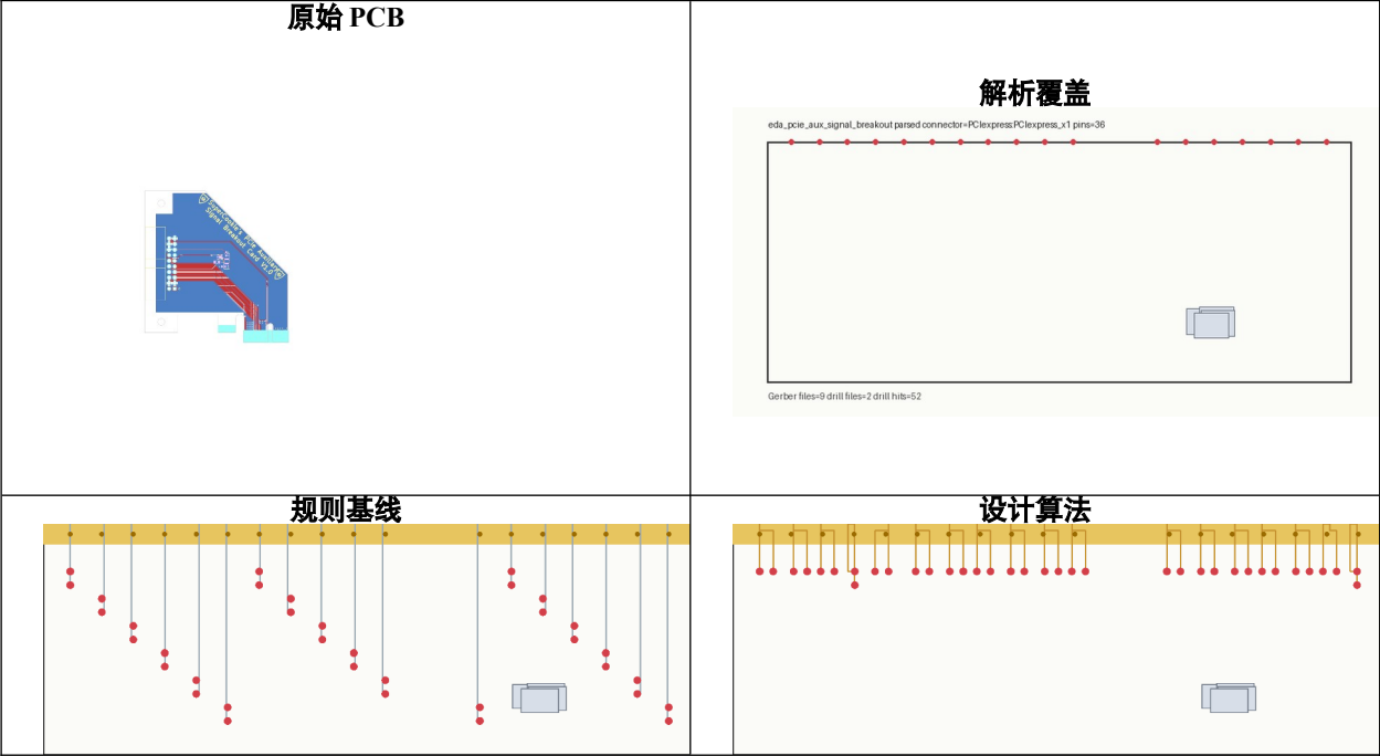
图 A-5 pcie aux signal breakout 案例独立截图对比
