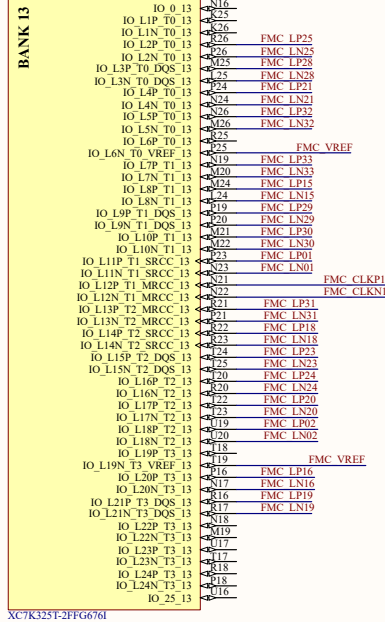
U1B
