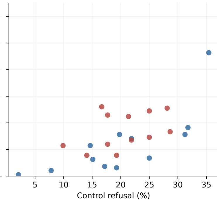
Disempowerment
