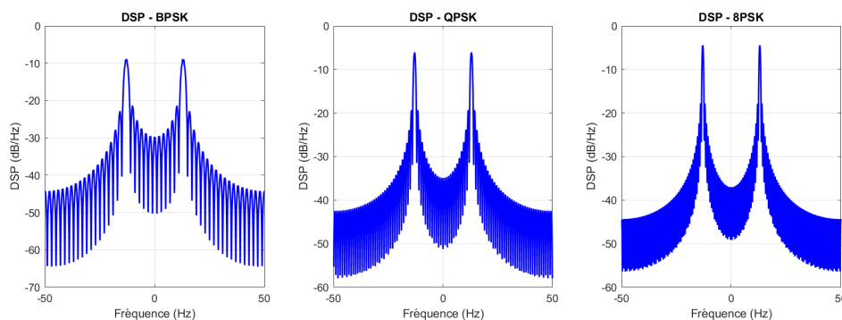
FIGURE 9 – Q23 : DSP des signaux modulés
