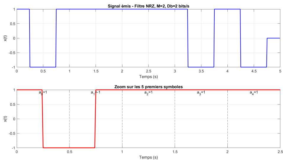
FIGURE 3 – Signal émis par l'émetteur complet
