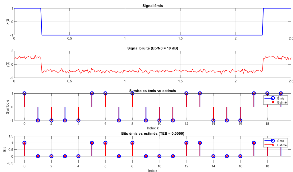
FIGURE 5 – Chaîne complète : émetteur, canal, récepteur
