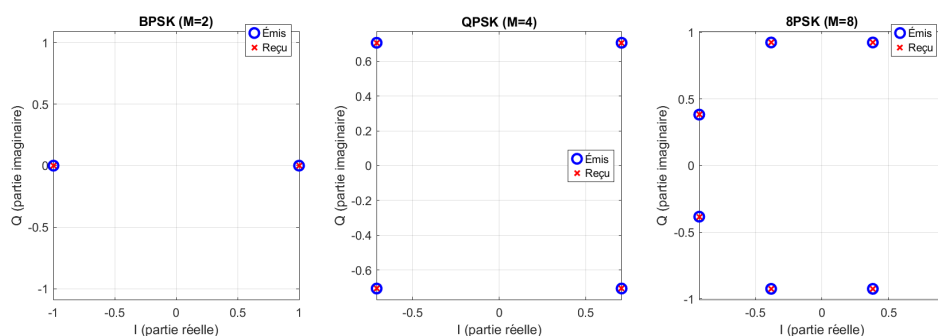
FIGURE 8 – Q22 : Symboles dans le plan complexe pour différentes modulations
