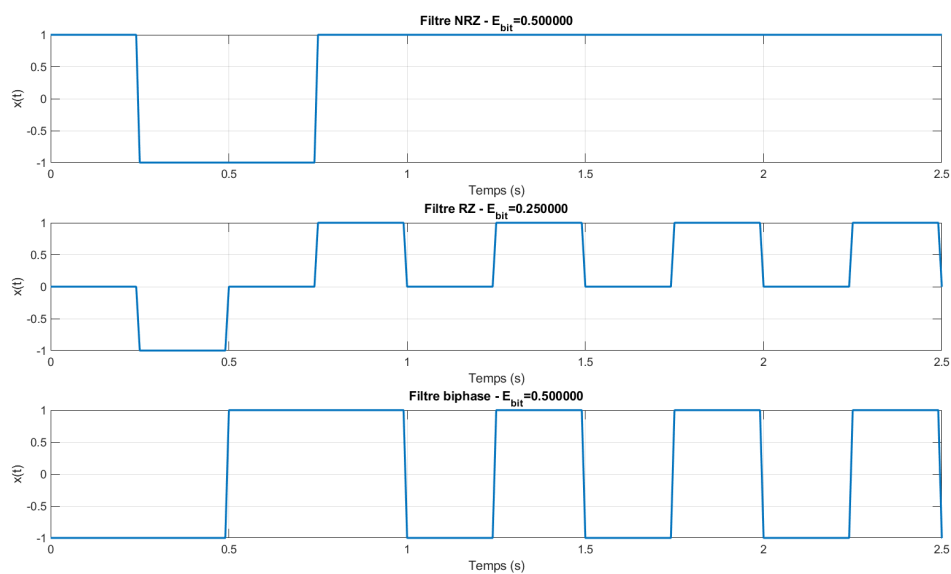
FIGURE 4 – Comparaison des signaux émis avec différents filtres
