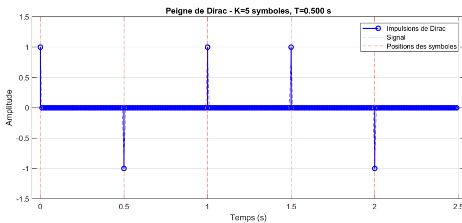
FIGURE 1 – Peigne de Dirac généré à partir d'une série de symboles
