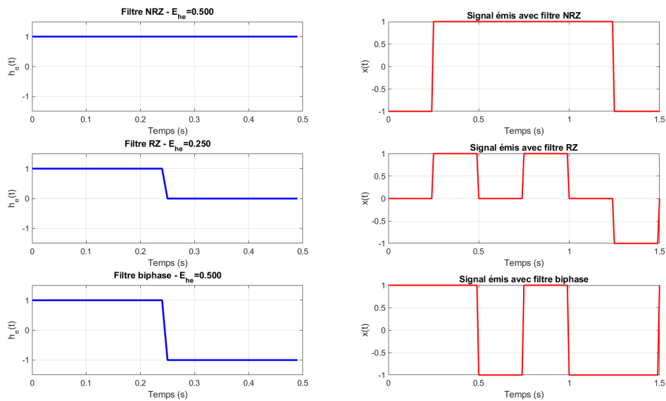
FIGURE 2 – Différents filtres de mise en forme et signaux émis correspondants
