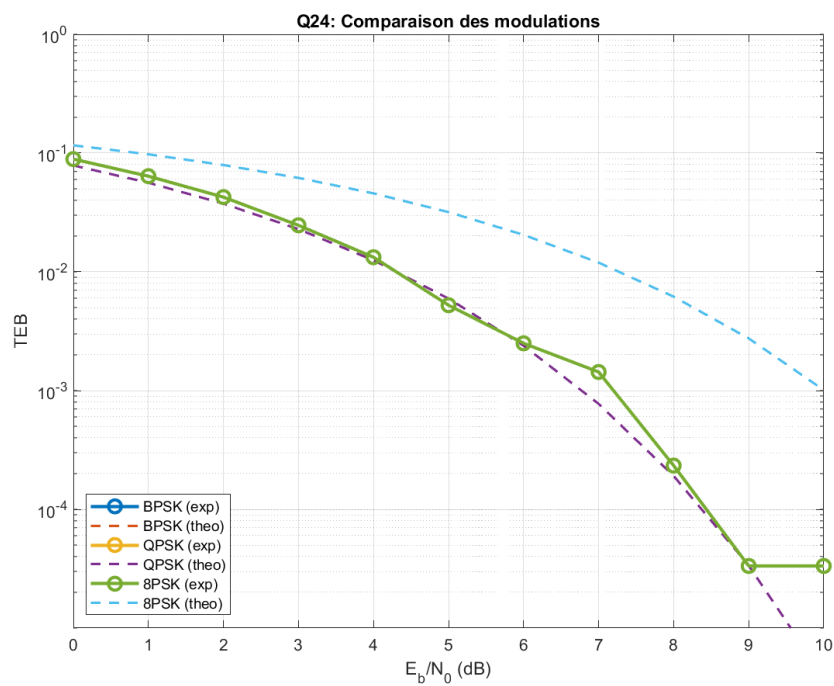
FIGURE 10 – Q24 : TEB des différentes modulations
