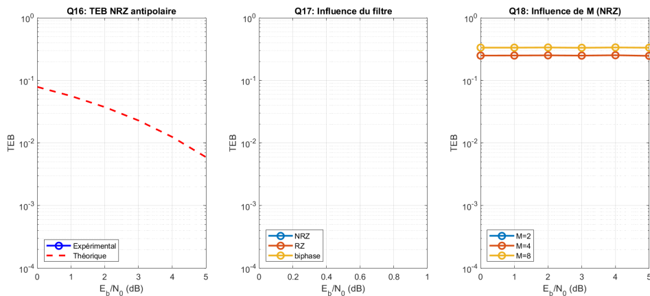
FIGURE 6 – Performances : TEB en fonction de E_b/N_0
