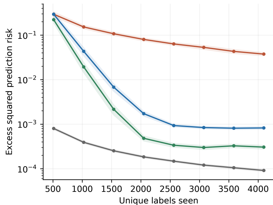
Noise SD 0.1
