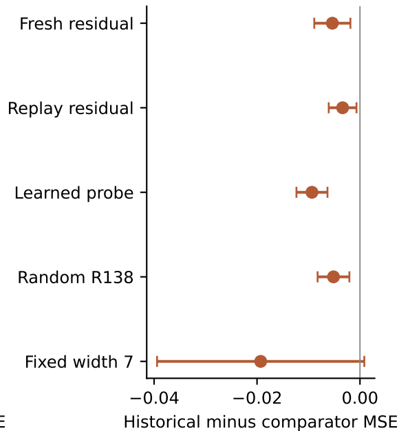
indefinite noisy
