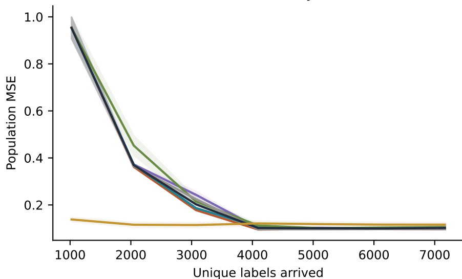
indefinite noisy
