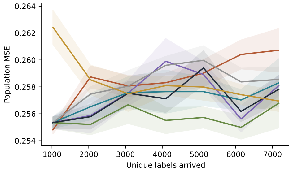
indefinite noisy
