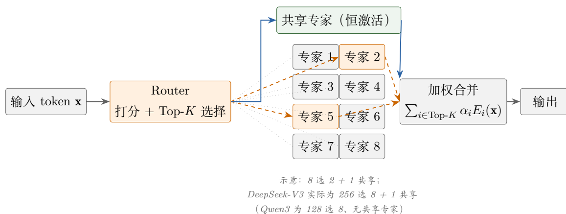
图 7: MoE 层工作机制：Router 为每个 token 打分并选出 Top- K 个专家，仅被选中的专家（橙色）参与计算，输出按门控权重 \alpha_i 加权合并；共享专家每 token 恒激活，负责“通用知识”。
