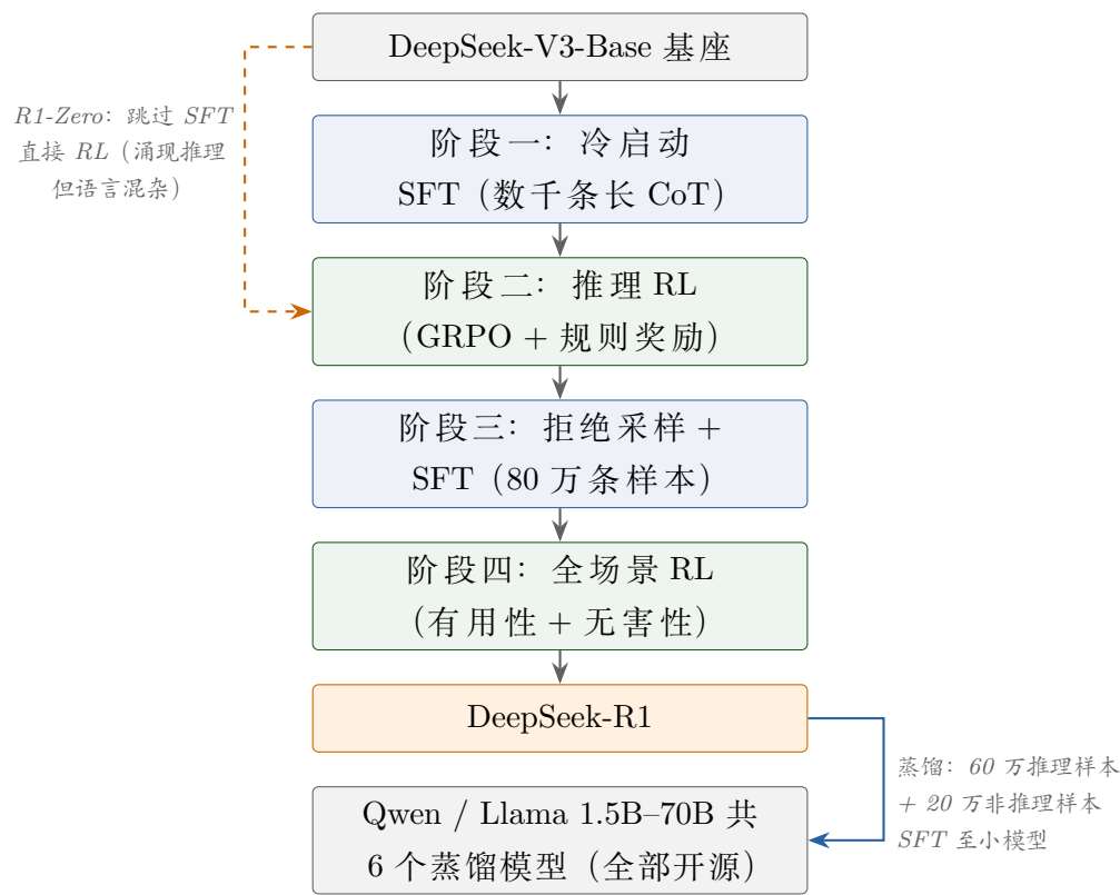
图 10: DeepSeek-R1 四阶段训练流水线：橙色虚线是 R1-Zero 的对照路径（验证“纯 RL 涌现推理”）；蓝色实线展示蒸馏路线——小模型无需自己跑 RL，直接继承 R1 的推理模式。
