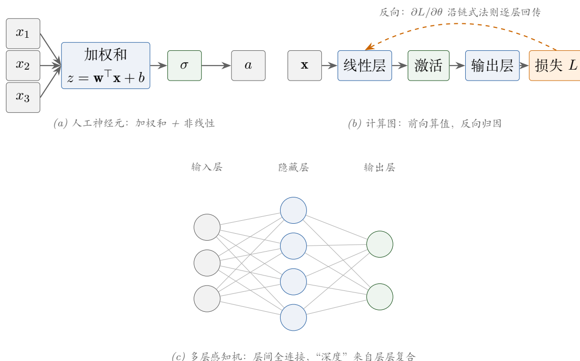
图 2: 深度学习的三个基本视图：(a) 人工神经元；(b) 计算图上的前向传播与反向传播；(c) 多层感知机——现代 LLM 就是把 (c) 的宽度与深度放大七个数量级、再把隐藏层换成注意力与 SwiGLU 的产物。
