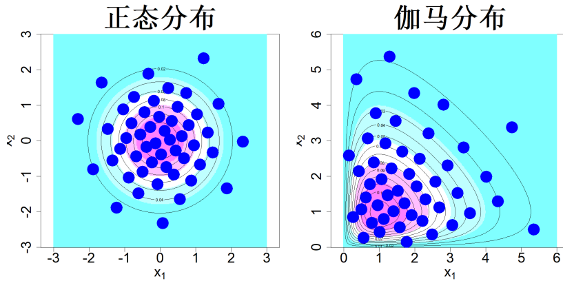
图 5.4： 通过均匀设计的逆概率变换得到的二元正态分布（左）与伽马分布（右）的 50 个代表点。图中同时展示了两种分布的图像与等高线
