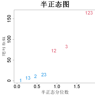
图 8.1: 不包含 x_4 的式 (8.3) 中模型绝对系数的半正态图
