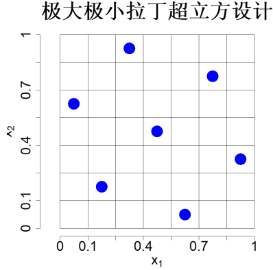
图 4.8: 7 点最大最小距离拉丁超立方设计
