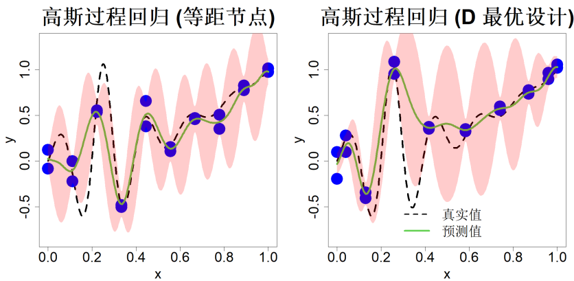
图 2.9： 采用 10 点等间隔设计点（左侧）与 10 点 D 最优设计点（右侧）并设置两组重复试验的高斯过程回归
