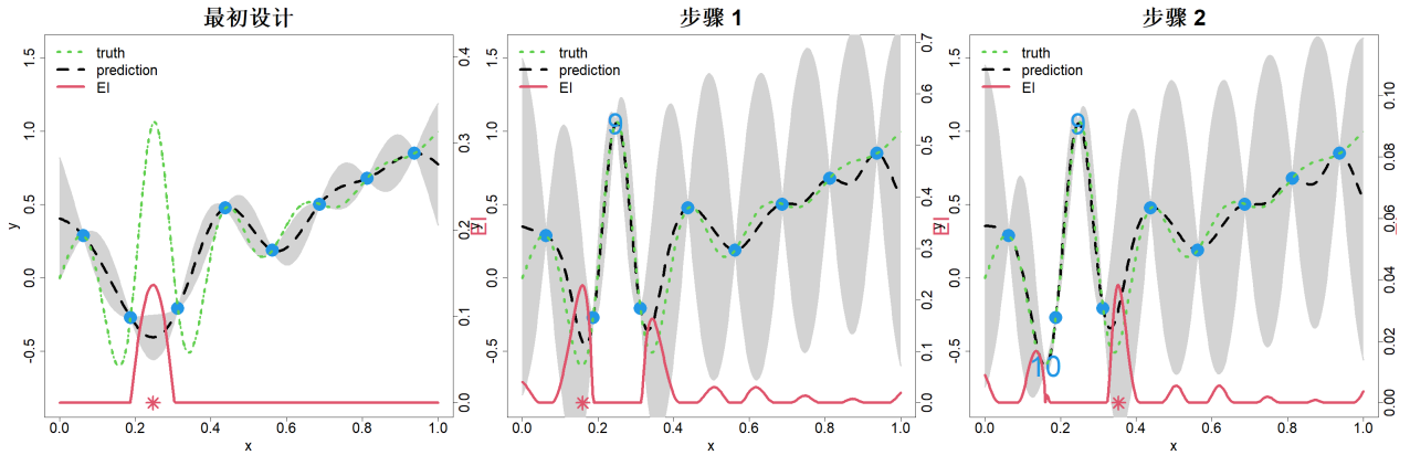
图 7.5：对式 (2.1) 中的一维函数执行期望改进最小化算法的两次迭代
