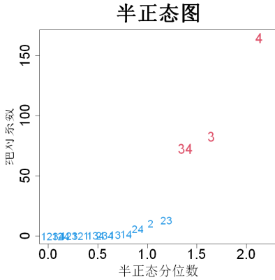
图 8.2： 式 (8.9) 中系数绝对后验均值的半正态图
