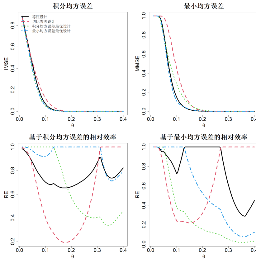
图 3.3： 图 3.2 中四种设计方案在积分均方误差（IMSE）与最小最大均方误差（MMSE）指标下的相对效率。将参数 \theta 固定为 0.1，即可求得分别适配积分均方误差、最小最大均方误差的最优设计方案
