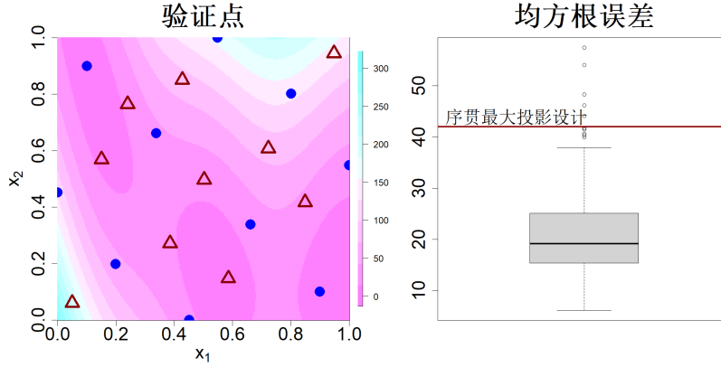
图 4.14: 左侧图像展示了马克斯普罗设计样本（蓝色圆点）与通过序贯马克斯普罗方法生成的验证点（红色三角形）叠加在布拉宁函数图像上的效果。右侧图像为 100 组随机验证集均方根误差的箱线图
