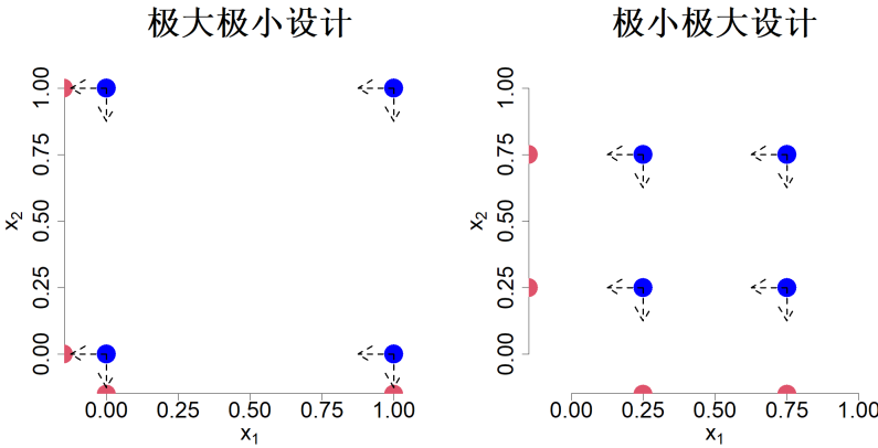
图 4.6：四轮试验下的极大极小与极小极大设计，及其在各坐标轴上的投影
