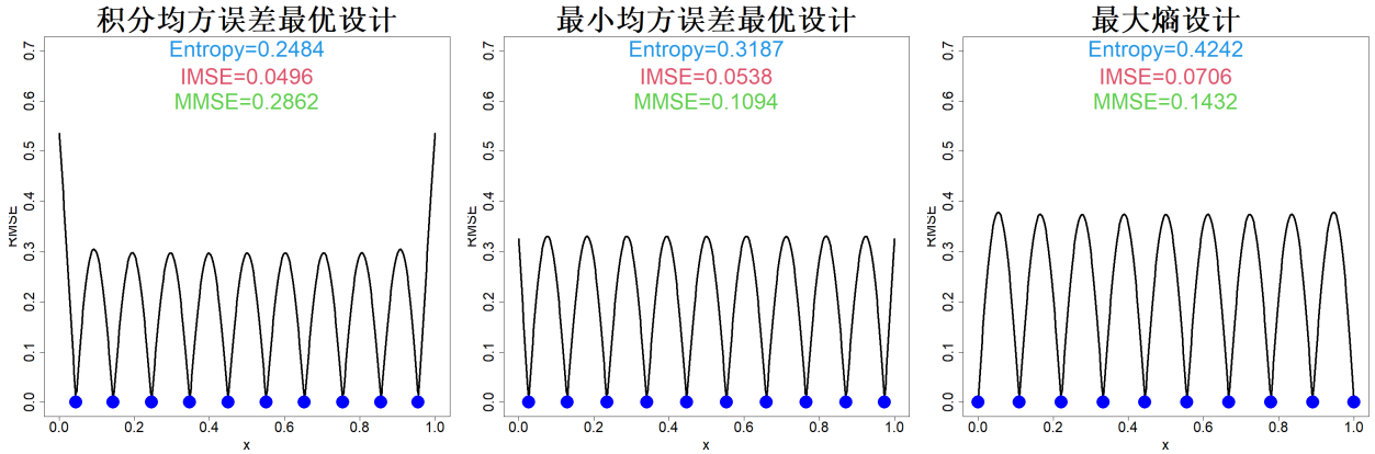
图 3.4: 在参数 \theta = 0.1 的条件下, 采用集成均方误差最优设计、最小均方误差最优设计与最大熵设计 (蓝色圆点)
