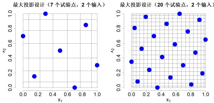
图 4.10：维度 p = 2 、样本量 n = 7 （左图）与 n = 20 （右图）对应的最大投影设计
