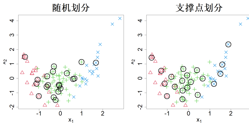
图 10.3： 通过随机采样（左侧）和支撑点划分（右侧）选取的测试点（圆形）。三种响应类别分别以红色三角形、绿色加号和蓝色叉号表示
