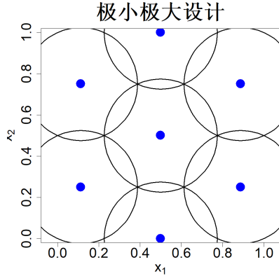
图 4.2: 7 点极小极大设计
