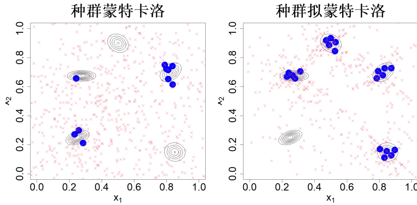
图 5.9: 该混合正态示例中，来自种群蒙特卡洛（左图）与种群拟蒙特卡洛（右图）的 800 个样本（红色叉号）以及最终的候选中心集合（蓝色实心圆）
