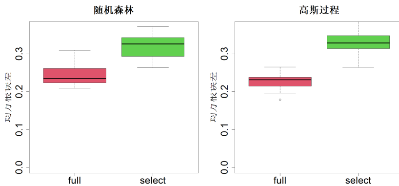
图 11.2: 采用全部八个预测变量，以及通过基于总指标的因子重要性排序与选择方法筛选得到的因子集，分别使用随机森林（左侧）与高斯过程（右侧），在混凝土数据集测试集上得到的均方根预测误差
