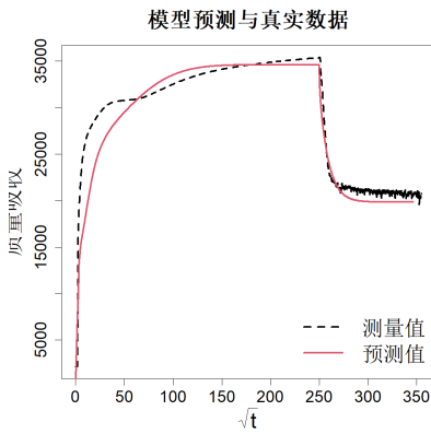
图 9.3：物理实验测得的质量吸附量与经校准的反应 - 扩散模型预测值
