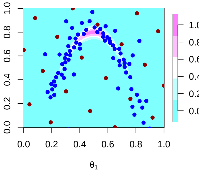
MED points with annealing
